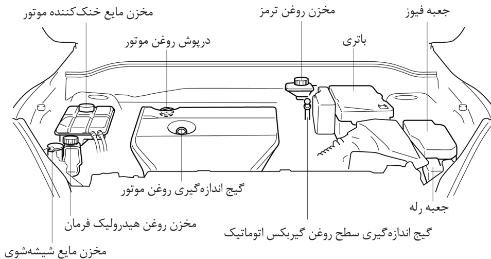
موتور 2.0 MZR
