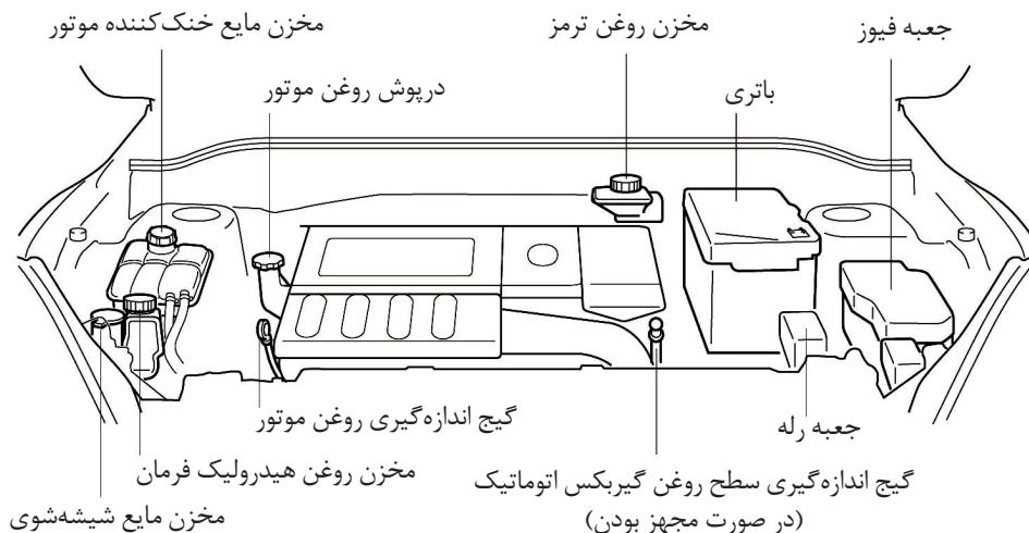
موتور 2.0 MZR
