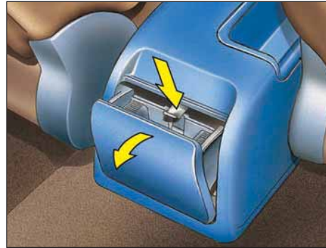
جاسیگار بها جهت خالی کردن آن، زبانه قفل را که در زیر آن قرار دارد کشیده و آن را بلند کرده و به طرف خود بکشید. نصب جاسیگاری جاسیگاری را در جای خود قرار داده و به طور کامل به داخل فشار دهید. در روی کنسول عقب در را پایین بیاورید. جهت خالی کردن، جاسیگاری را به طرف خود کشیده و همزمان زبانه قفل آن را به پایین فشار دهید.
